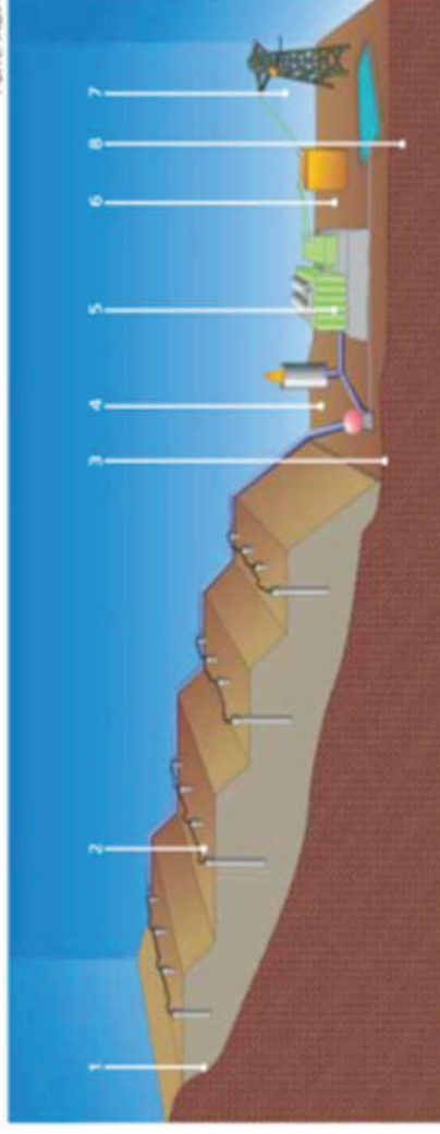
Esquema del sistema de recuperació del biogàs en el dipòsit controlat del Garraf
